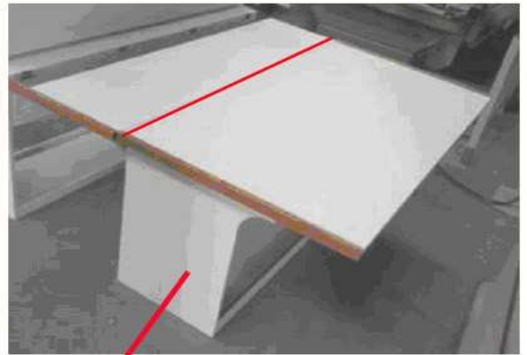
Nuovo unico tavolo centro dinette con anta mobile (lato sx) Rifiniture spigoli tavolo dinette in teck
